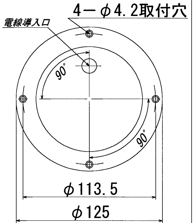
<<取付面 寸法図>>
