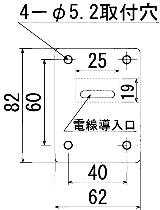
<<取付面 寸法図>>
