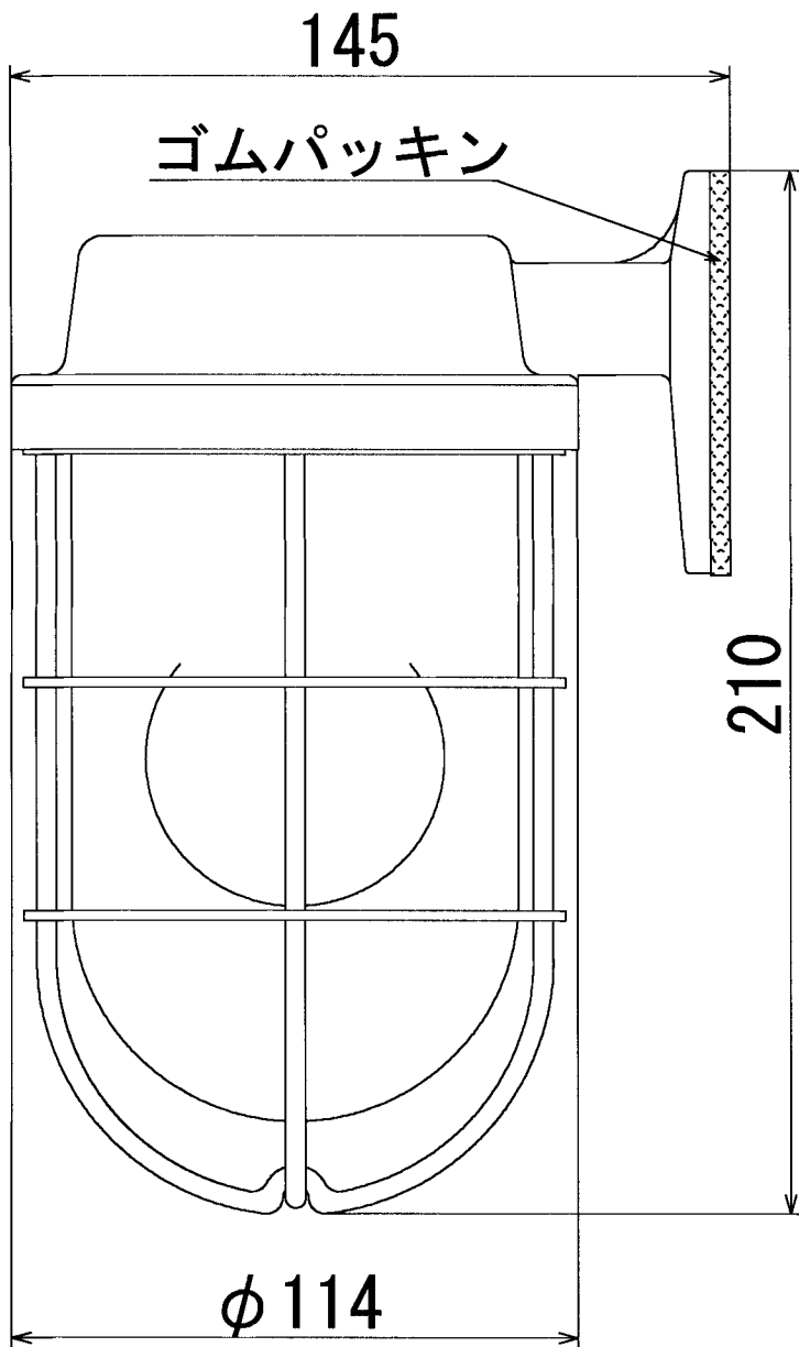
<<取付面 寸法図>>
