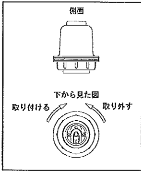
■締付リングの 取り付け取り外しかた
