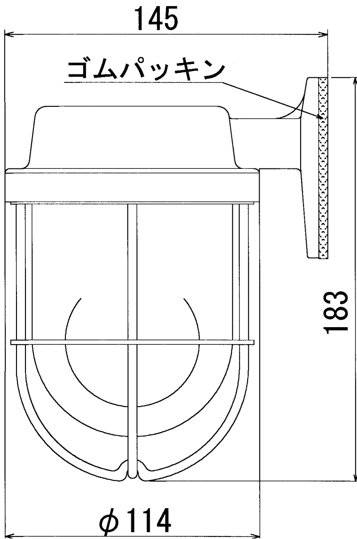
<<取付面 寸法図>>
