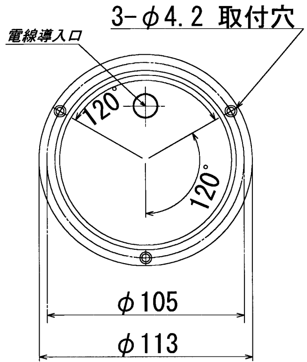
<<取付面 寸法図>>
