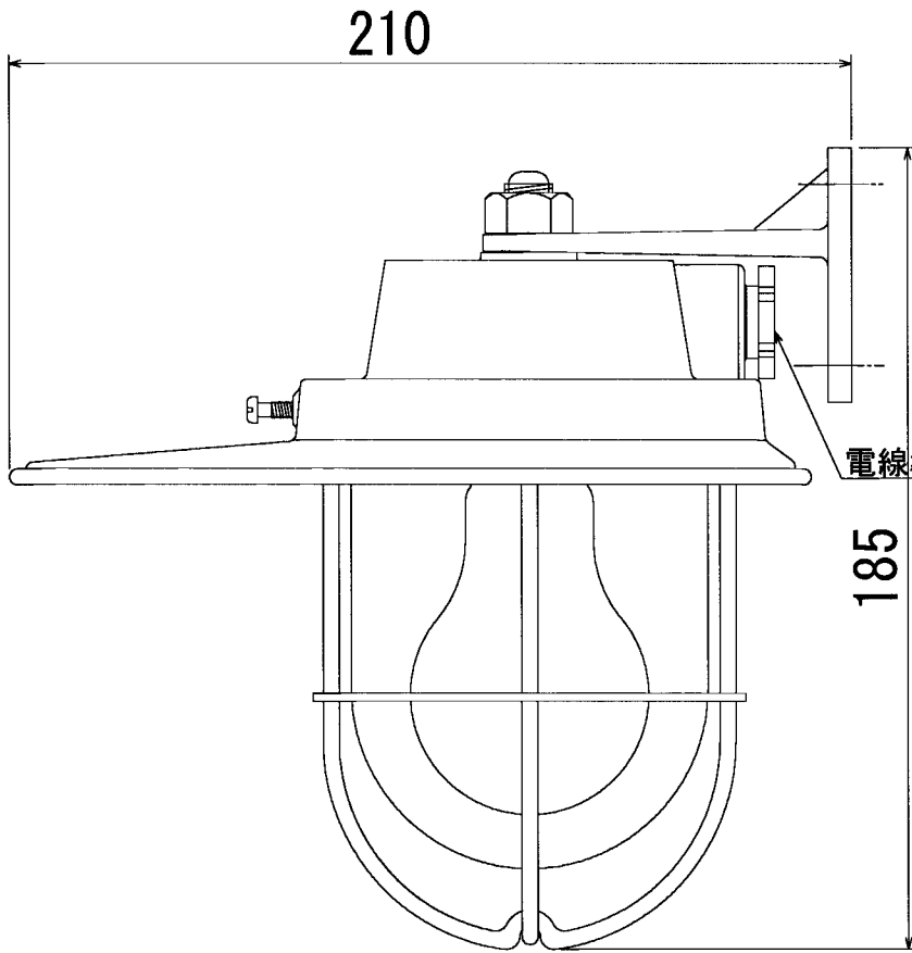
<<取付面 寸法図>>
